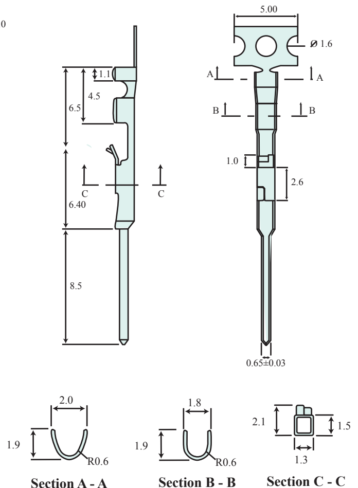
MMWCA系列 散离线压接公端子
